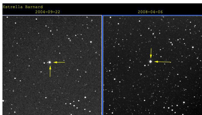
Moviment de l'estrella de Barnard 2004-8. R. Naves
